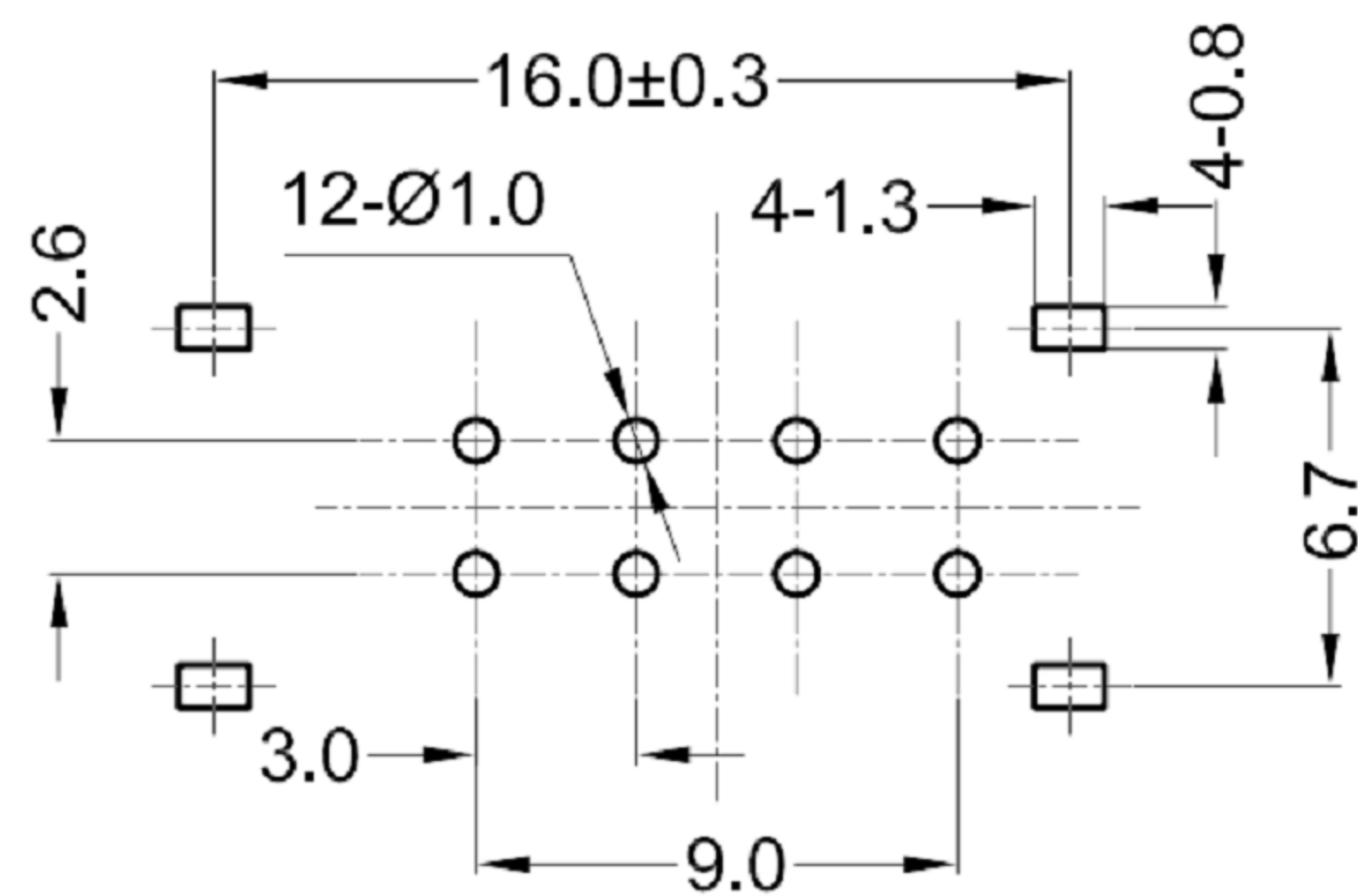
P.C.B LAYOUT
